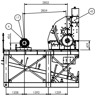
SECCIÓN B-B ESCALA 1 : 75
