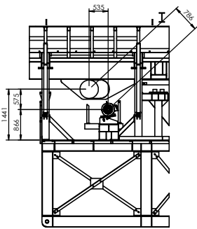
SECCIÓN C-C ESCALA 1 : 75
