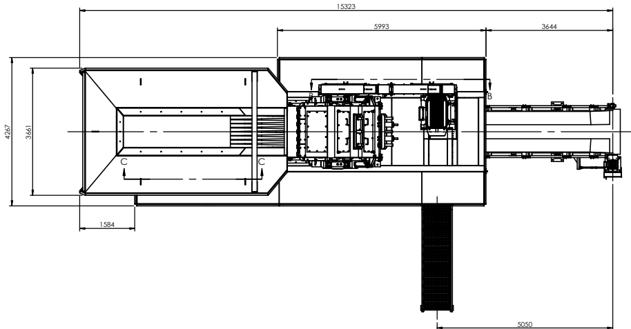
VISTA PLANTA
